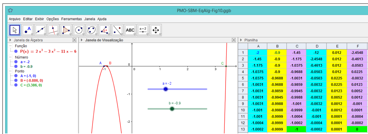
Figura 10: Cálculo da raiz de 2x^3 - 3x^2 - 11x - 6 = 0 no GeoGebra, utilizando a = -2 e b = -0,9 .
