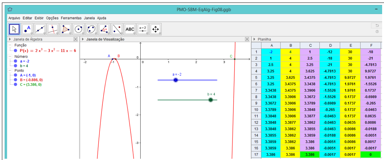
Figura 8: Cálculo da raiz de 2x^3 - 3x^2 - 11x - 6 = 0 no GeoGebra, utilizando a = -2 e b = 4 .
