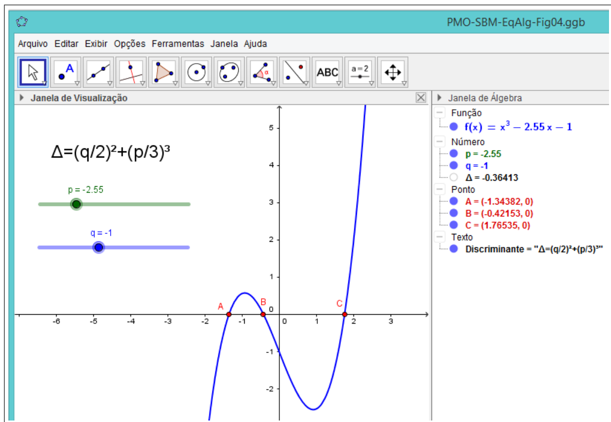
Figura 4: Caso \Delta < 0 .
