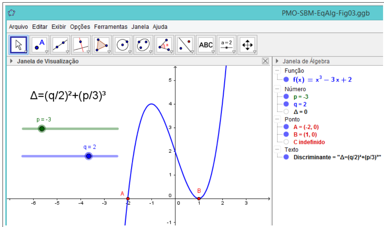
Figura 3: Caso \Delta = 0 .
