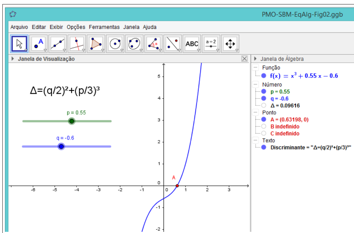
Figura 2: Caso \Delta > 0 .
