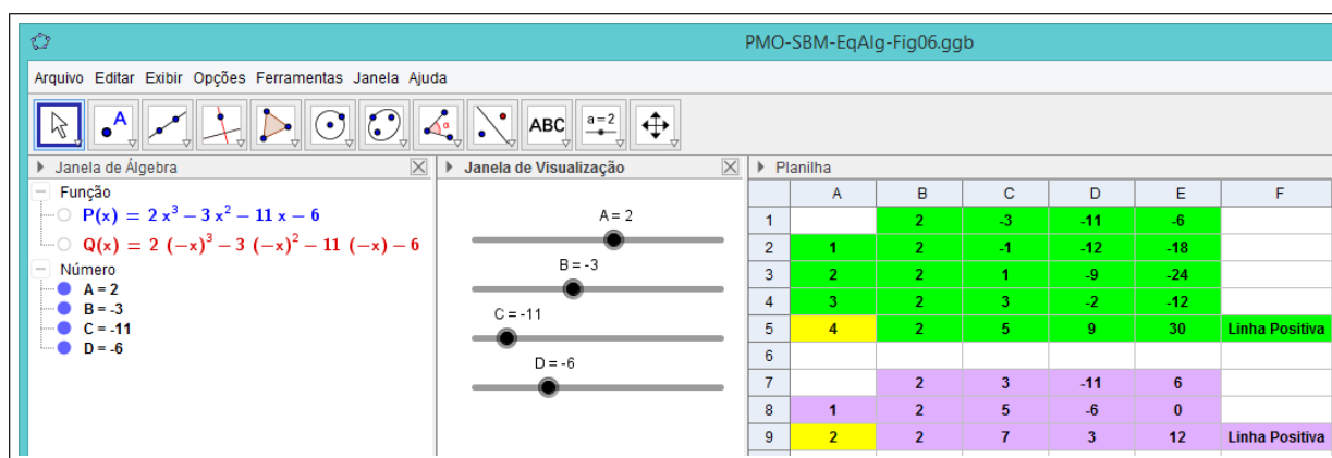
Figura 6: Cotas para as raízes da equação 2x^3 - 3x^2 - 11x - 6 = 0 .
